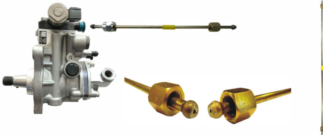
Tubería de banco de prueba para Common Rail de rampa a bomba
